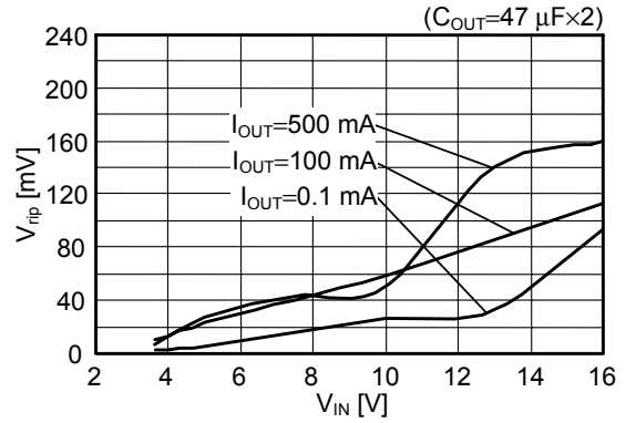
(4) S-8521B30MC
