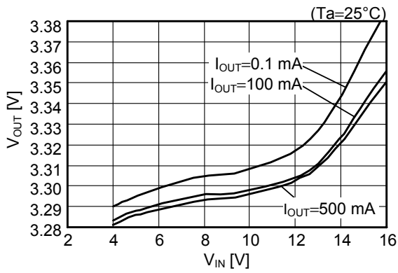
S-8521F33MC
