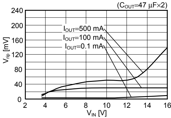
(3) S-8520B30MC
